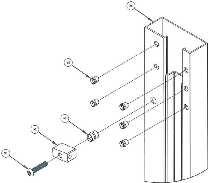
JAMB ASSEMBLY
